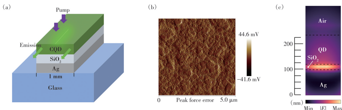
图 1 (a)Spaser 器件结构示意图;(b)CQD 薄膜的原子力显微镜图;(c)模拟的混合模式电场强度分布图
