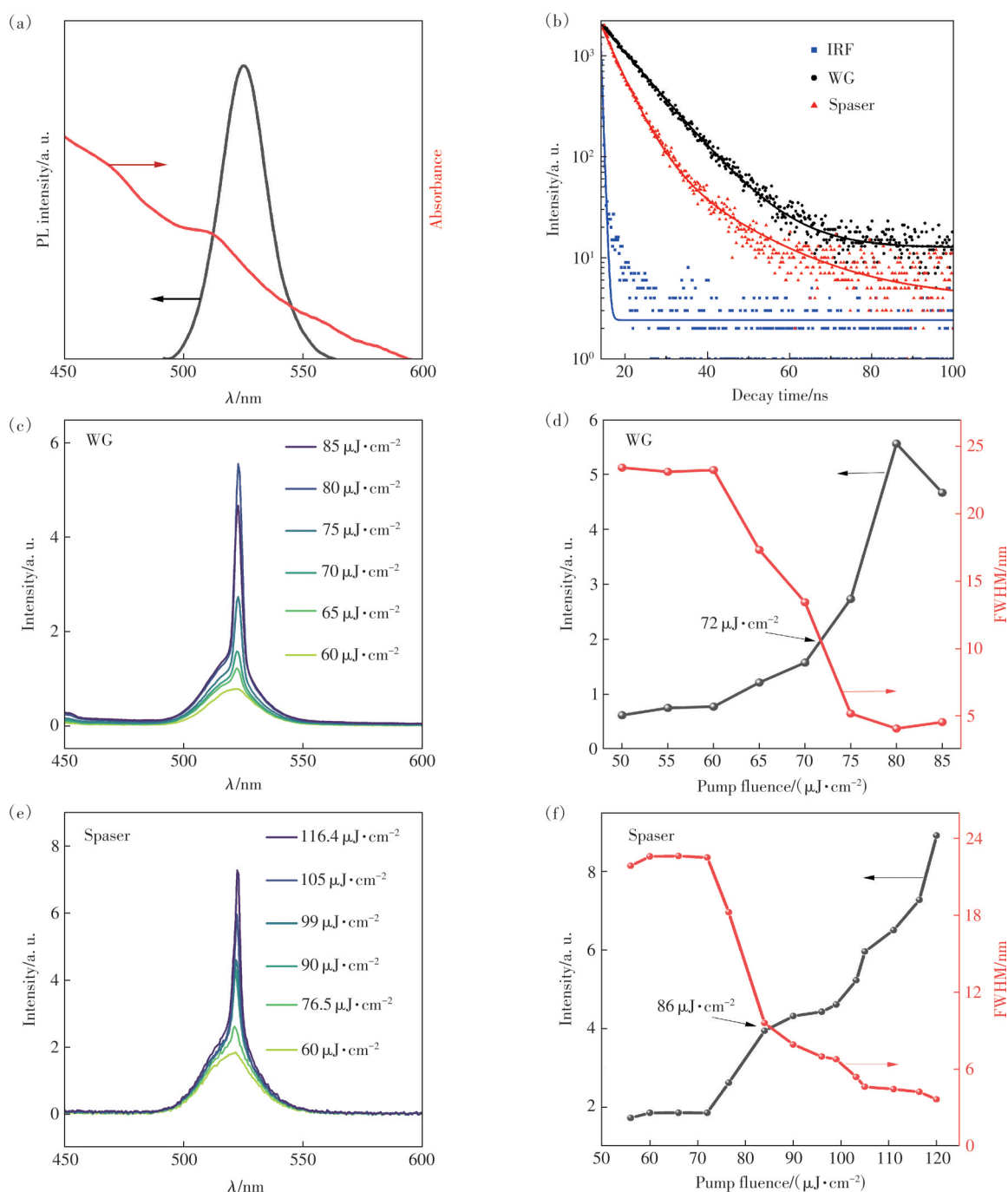
图2 (a)量子点材料PL及吸收光谱;(b)WG与Spaser样品的时间分辨PL衰减动力学;(c)不同泵浦能量密度下的WG样品边发射输出光谱;(d)WG样品的输出光强度和FWHM随泵浦能量密度的变化;(e)不同泵浦能量密度下的Spaser样品边发射输出光谱;(f)Spaser样品的输出光强度和FWHM随泵浦能量密度的变化
